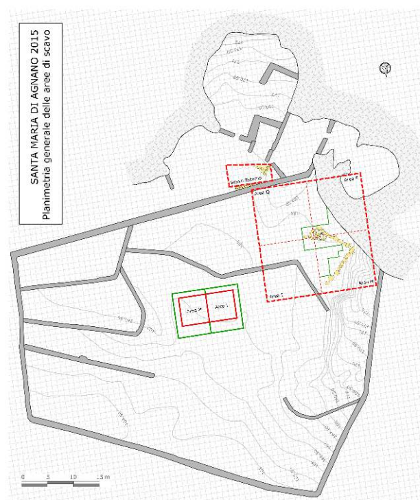
Figure 1 – Planimetria generale del sito con le aree di scavo indagate nel 2015.
